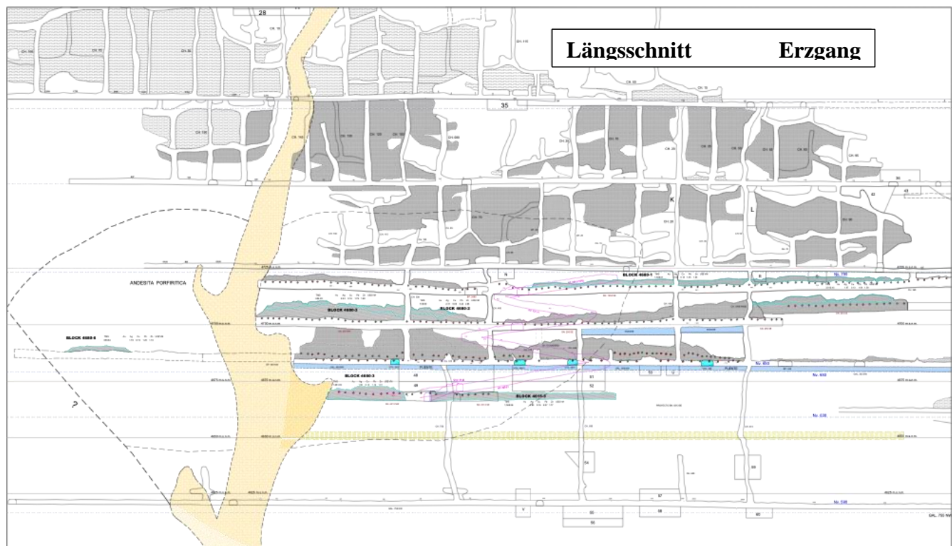
Abbildung 2: Längsschnitt des Erzgangs Tangana 1 - die im Monat Juli erschlossenen Stollen mit Erzförderung sind hellblau dargestellt.
