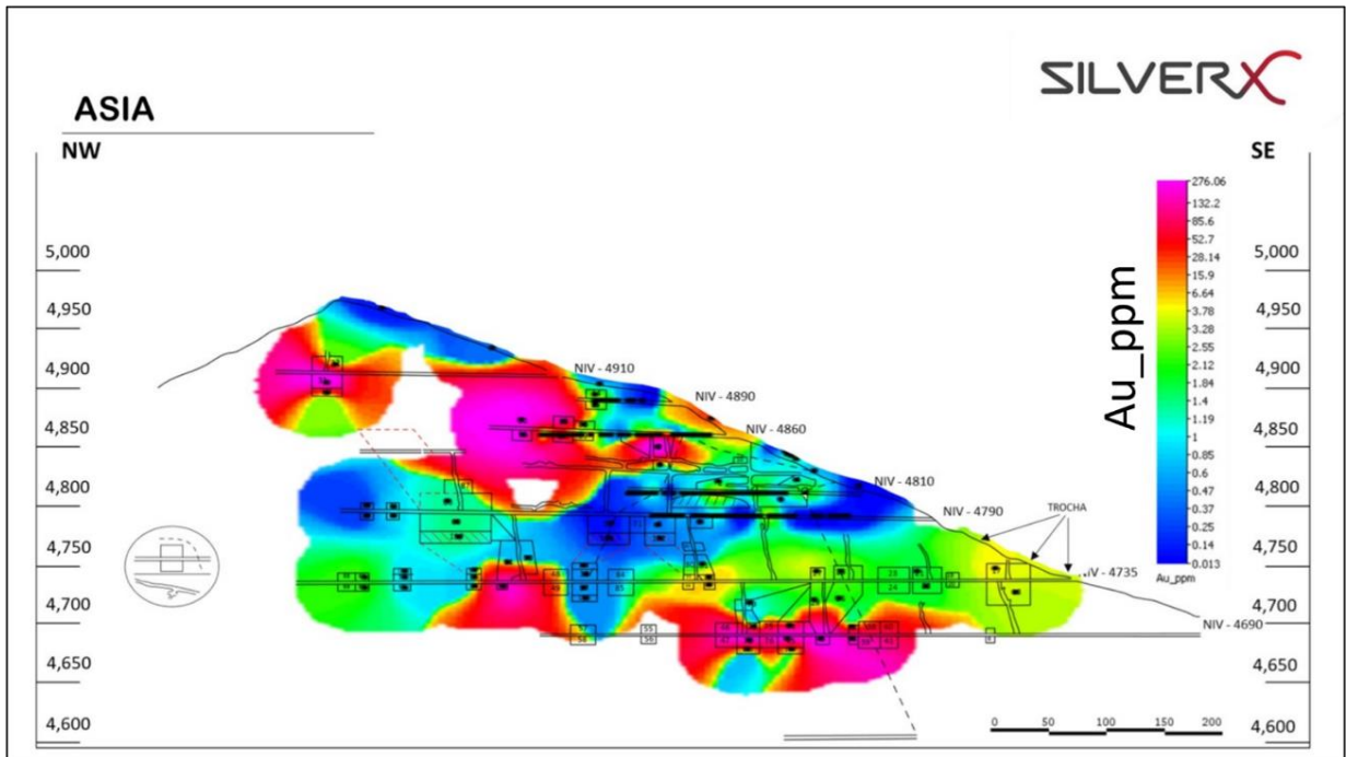
Abbildung 4: Isopachen der Au-Gehaltsschätzung im Längsschnitt des Erzganges Asia, Blickrichtung Norden. Die violetten und roten Bereiche markieren Gebiete mit erhöhten Goldgehalten, die aus historischen und aktuellen Probenahmen stammen.
