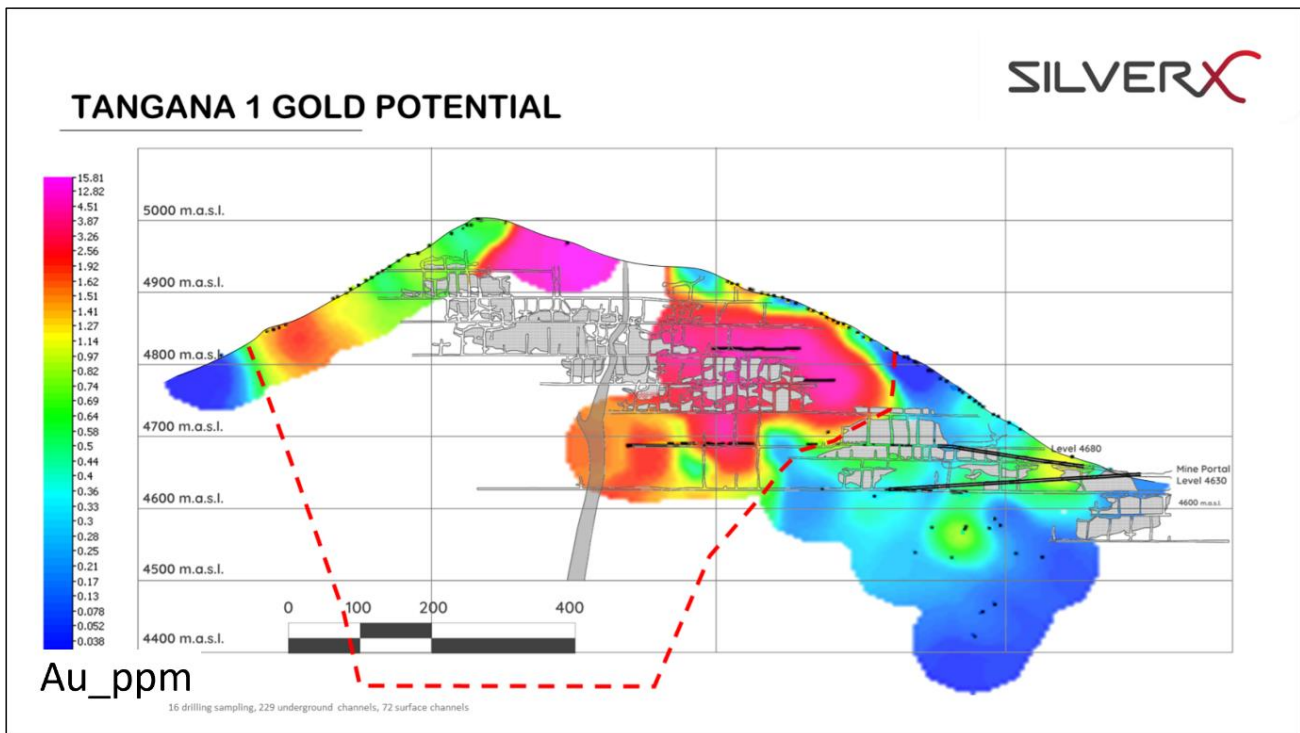
Abbildung 3: Isopachen der Au-Gehaltsschätzung im Längsschnitt des Erzganges Tangana 1, Blickrichtung Norden. Die lilafarbenen und roten Bereiche markieren Gebiete mit erhöhten Goldgehalten, die aus dem aktuellen Bergbau, Oberflächenproben und Bohrergebnissen stammen.
