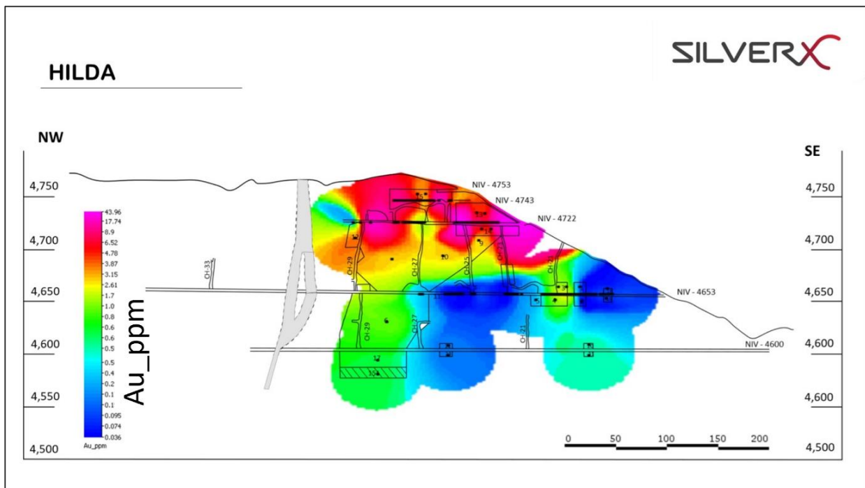
Abbildung 5: Isopachen der Au-Gehaltsschätzung im Längsschnitt des Erzganges Hilda, Blickrichtung Norden. Die violetten und roten Bereiche markieren Gebiete mit hohen Goldgehalten, die aus historischen und aktuellen Probenahmen stammen.
