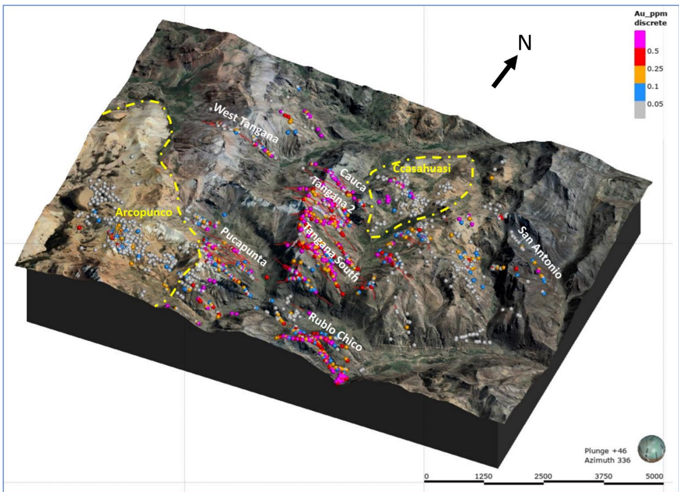
Abbildung 2: Isometrische Ansicht der Bergbaueinheit Tangana mit Lage der ausgewählten Goldproben und goldhaltigen Intrusionen, gelbe Umrandung.
